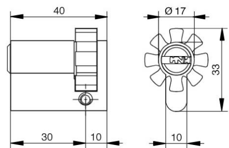
8-fach verstellbarer Schließbart
